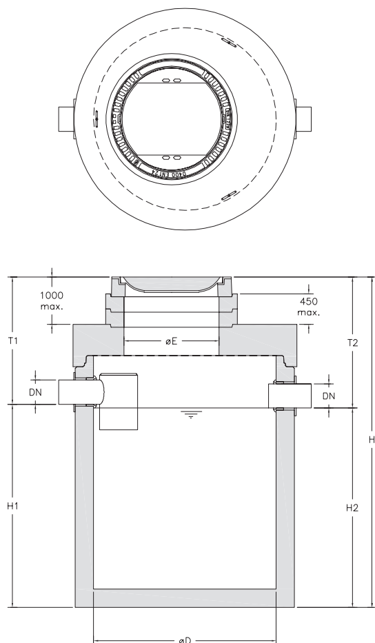
Afbeelding 4. Maattekening separate slibvang
