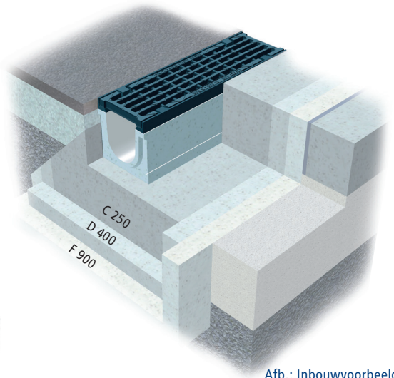
Afb.: Inbouwvoorbeeld
