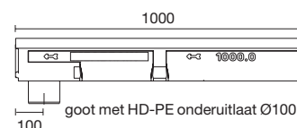
AQUAFIX V1000 met kitvoeg EN 1433
