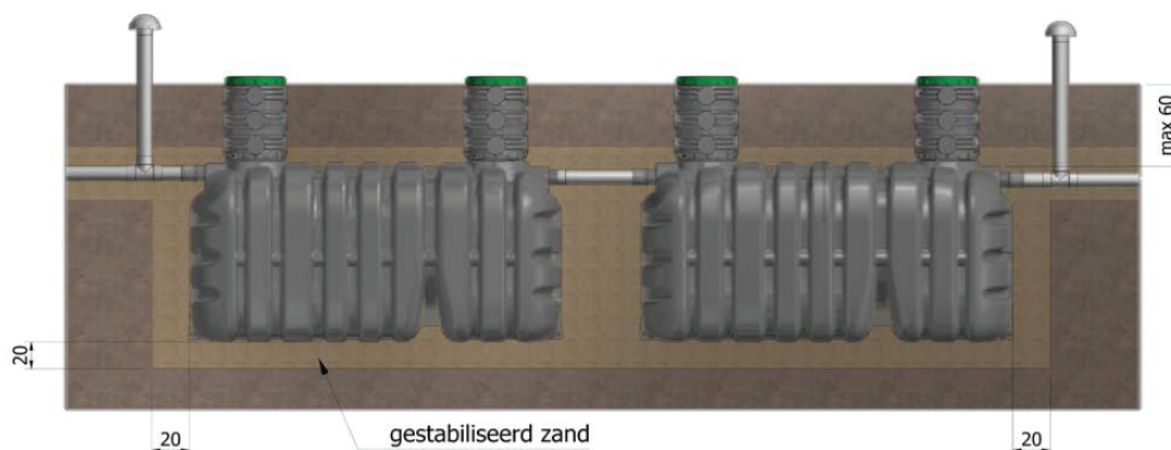
Inbouwtekening groenzone (maten in cm)
