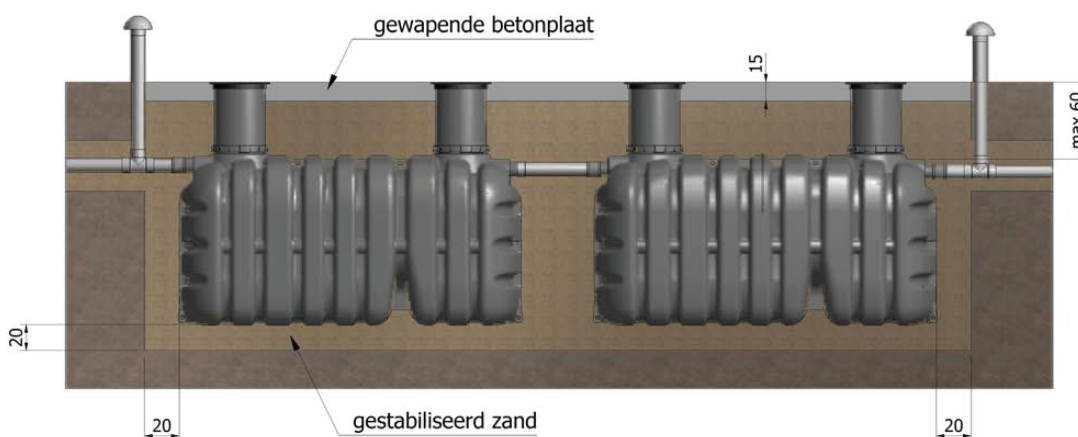
Inbouwtekening oprijt verkeerklasse B125 kN (maten in cm)
