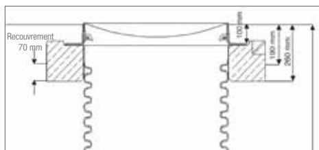
Betonnen verdeelplaat met kader en buffer
