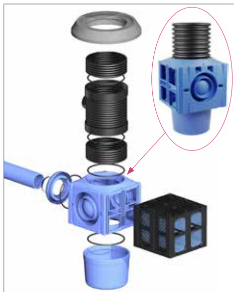
Zicht op de onderdelen van Sikkofix C3
